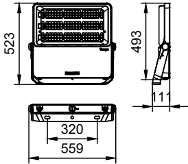
BVP433 LED465/CW 220~240V 345W SWB GC
